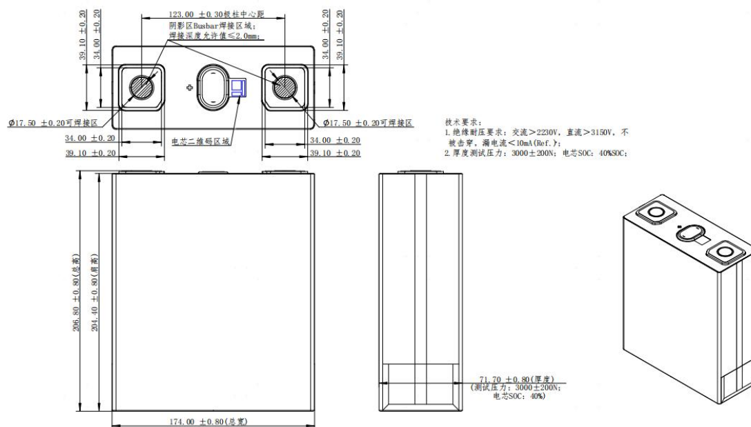
图 7.1 电池尺寸/mm
